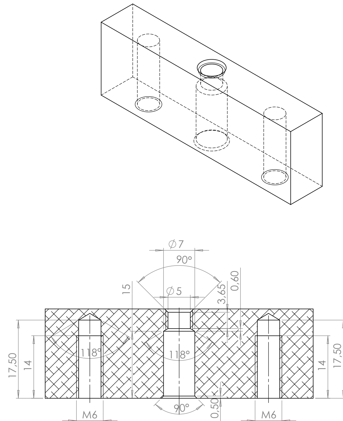
SECTION A-A
